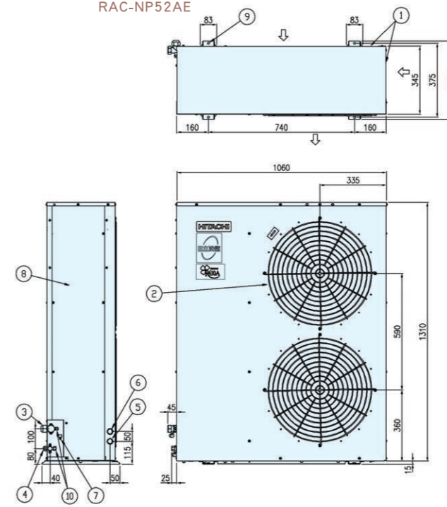
室外機 RAC-NP52A RAC-NP52AE
