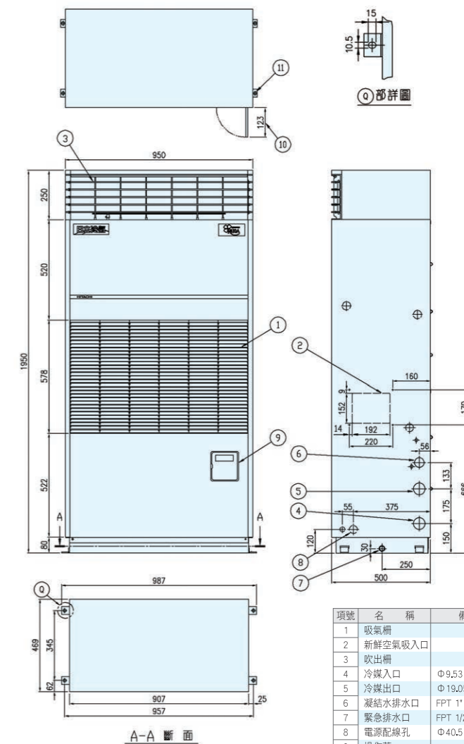
室內機 RPS-NP52A RPS-NP52AE
