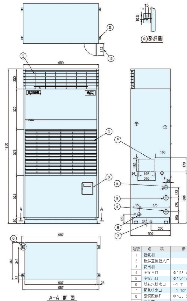
室內機 RPS-NP52AB
