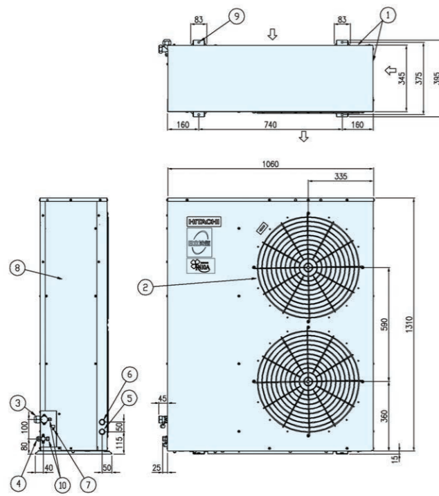
室外機 RAC-NP52AB
